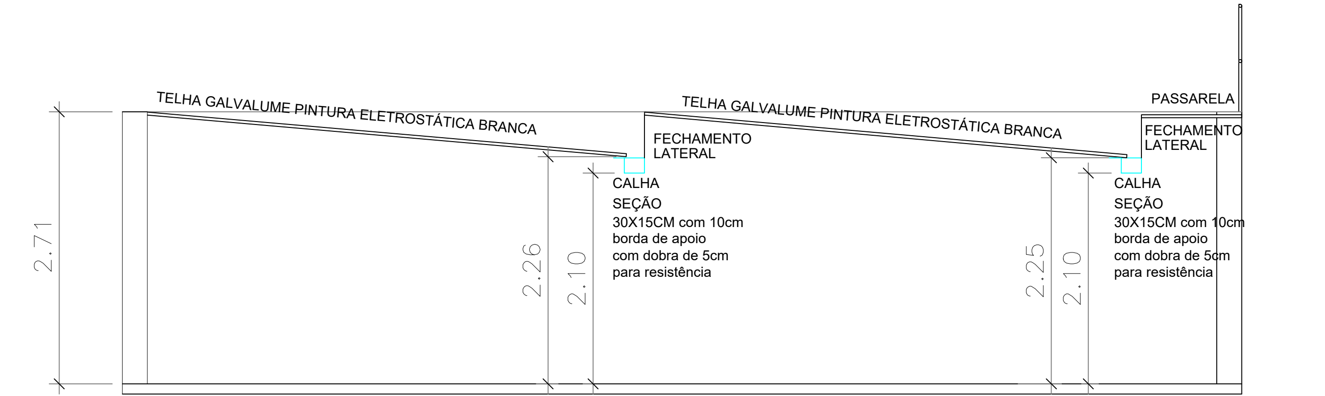
CORTE
