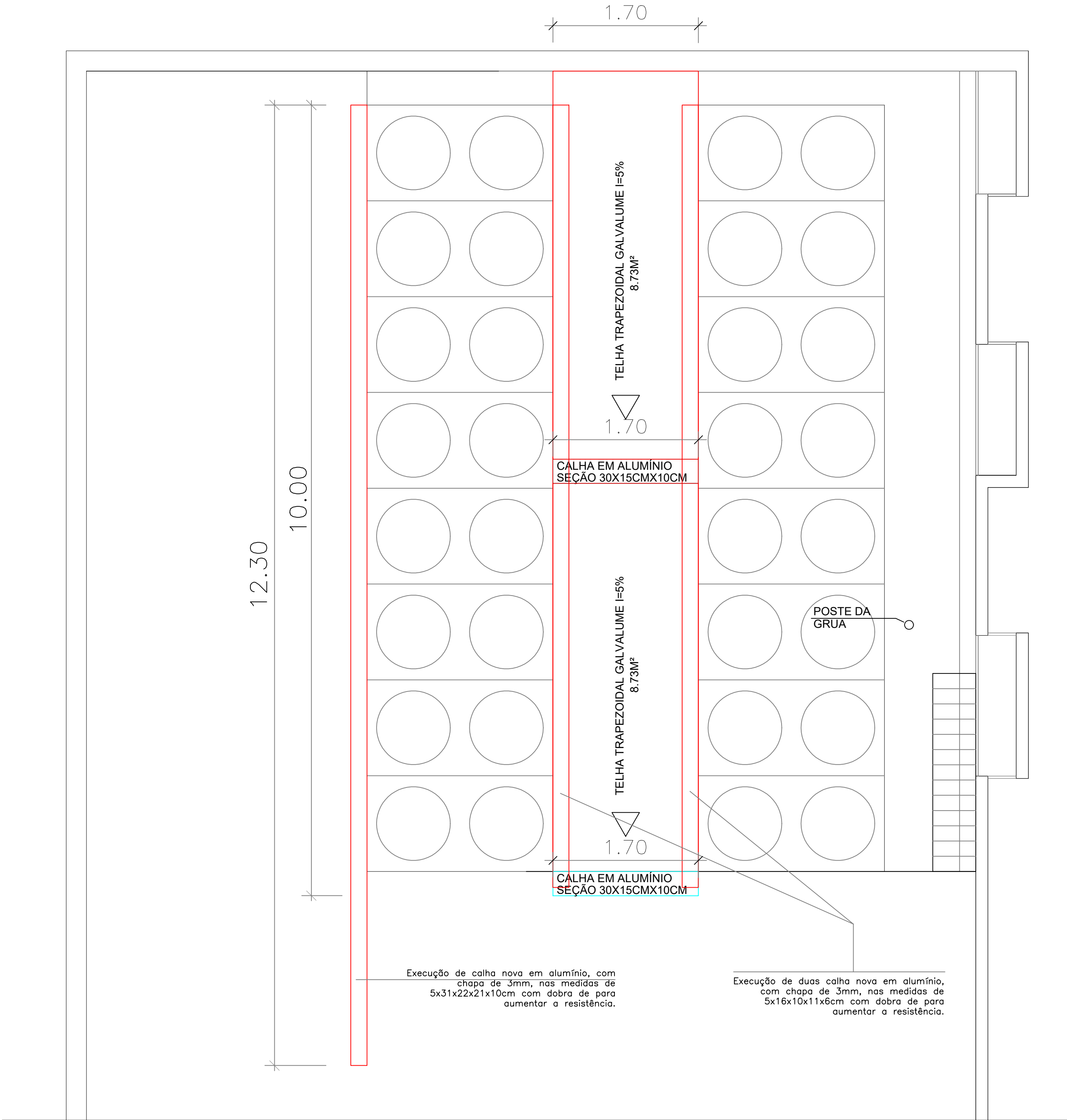
PLANTA BAIXA
